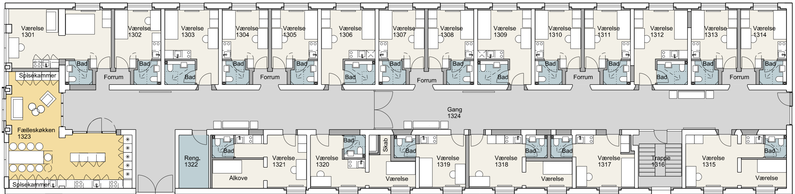
Plan, etage 3
